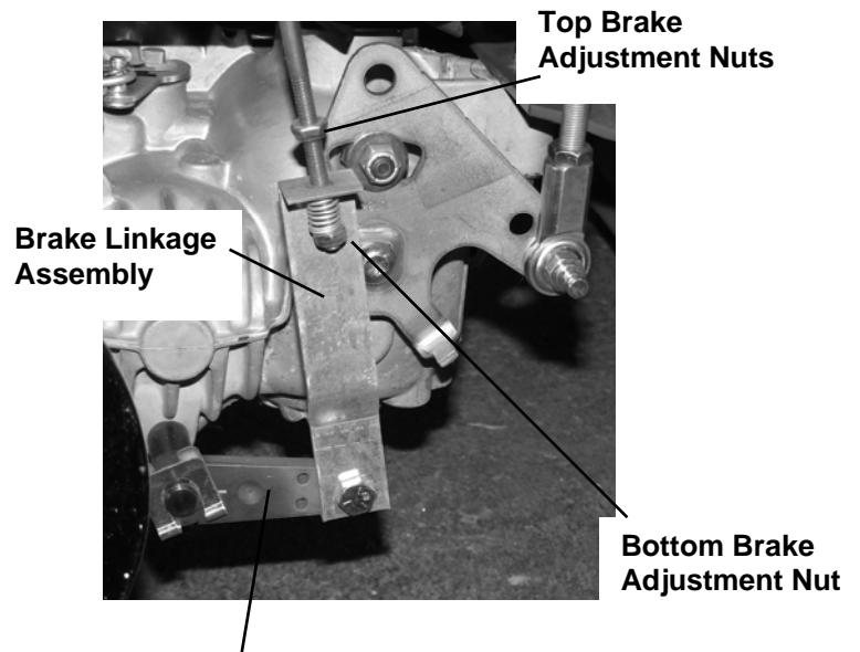
Brake Rod Arm
